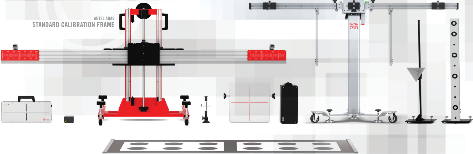
AUTEL ADAS MAG00 CALIBRATION FRAME
